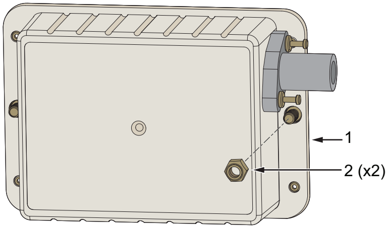
Figure 7: EHT Module
